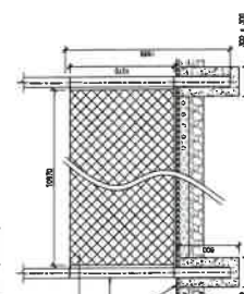
TENNIS NET DETAILS (N.T.S.)
